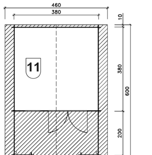
Angaben in cm
